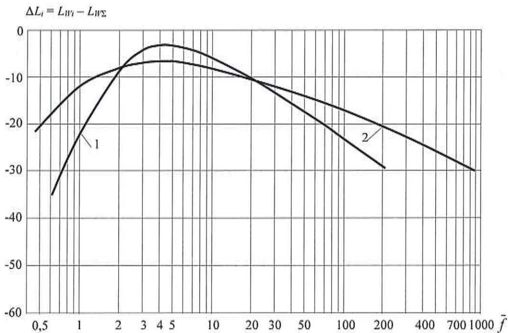
Рисунок 6.12 – Безразмерные частотные характеристики решеток
