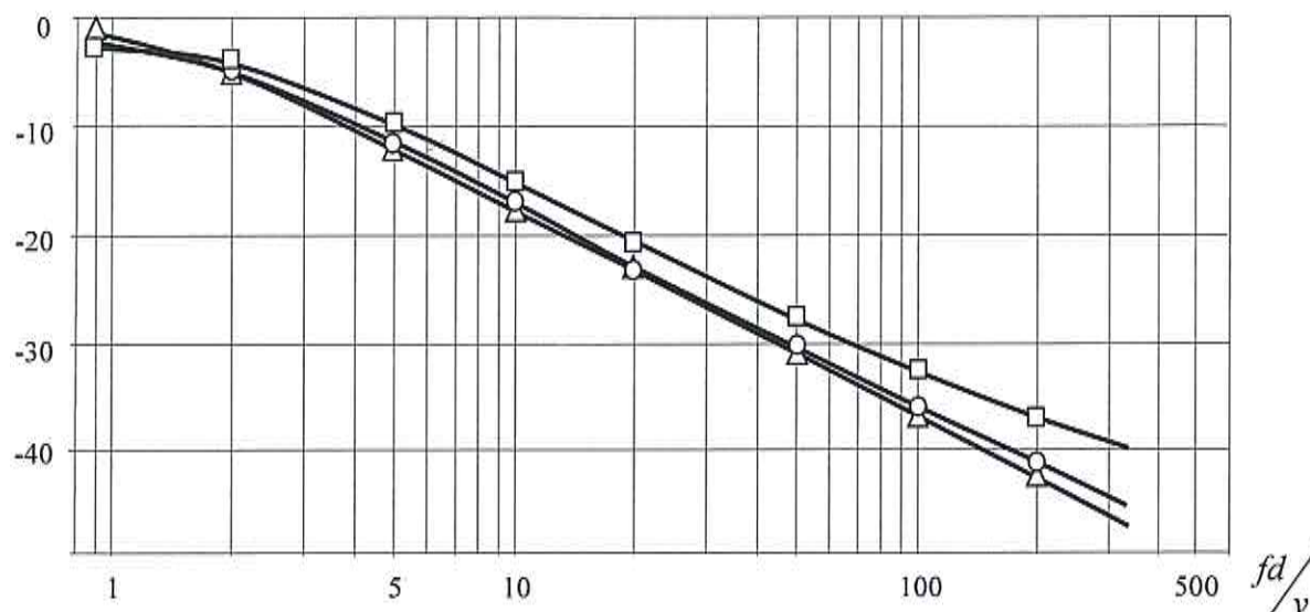
Рисунок 6.2 – Безразмерная частотная характеристика прямых участков воздуховодов разных сечений
