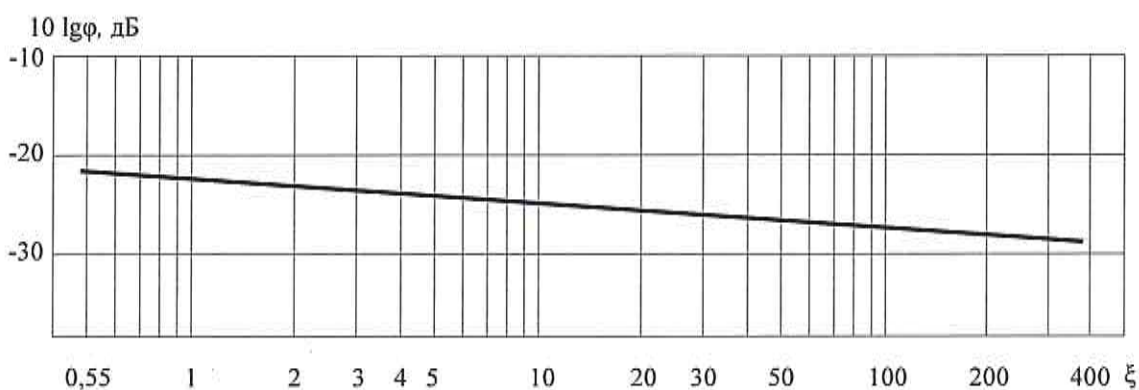
Рисунок 6.10 – Зависимость 10 \lg \phi от коэффициента местного сопротивленияшибера или дроссель-клапана
