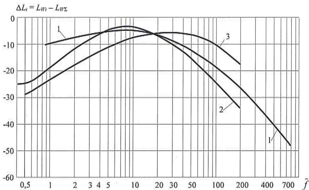
Рисунок 6.12 – Безразмерные частотные характеристики решеток
