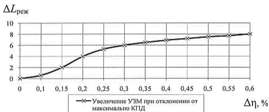
Рисунок 6.1 – Поправка \Delta L_{\text{реж}} на режим работы вентилятора
